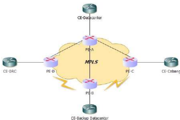
Gambar 4. Desain Konfigurasi Routing OSPF
