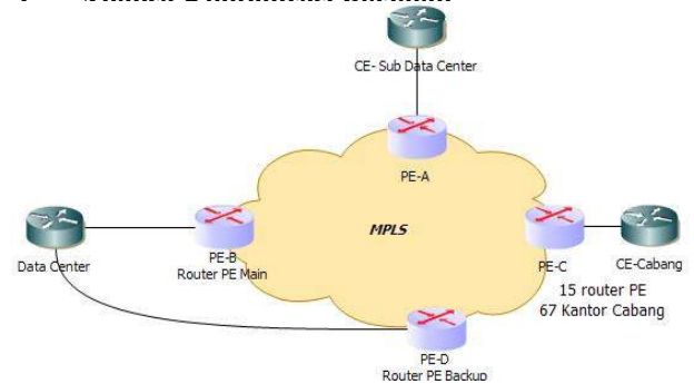
Gambar 3. Konfigurasi Jaringan
